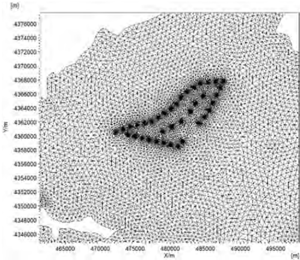
图 5.1.1-3 风电场工程区附近局部网格图
