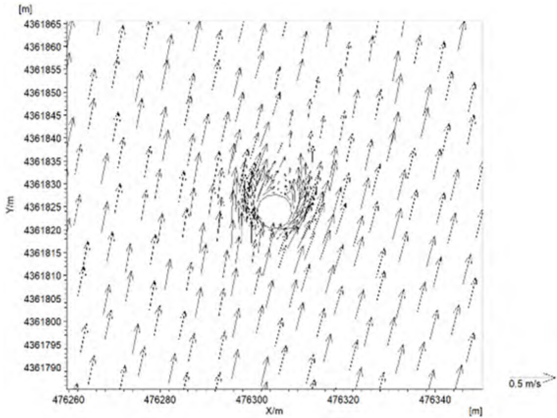
图 5.1.4-3 单个风电桩基局部涨急流场图
