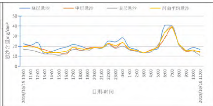
图 4.3.1-45 4#站秋季大潮期悬沙含量变化曲线图
