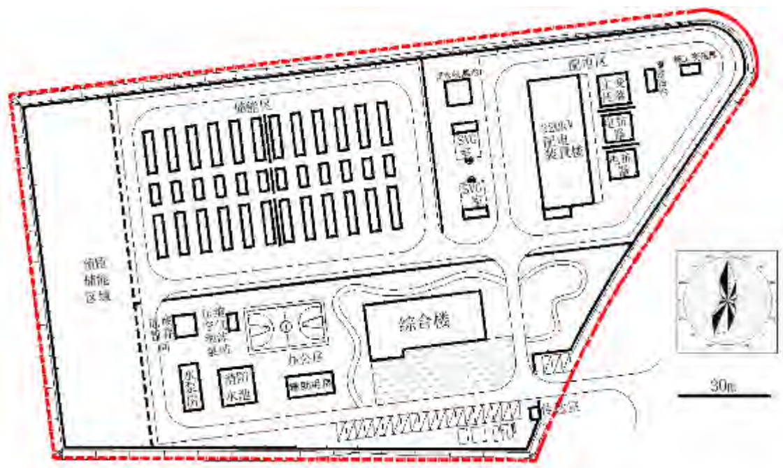
图 3.1.3-4 陆上集控中心平面布置图
