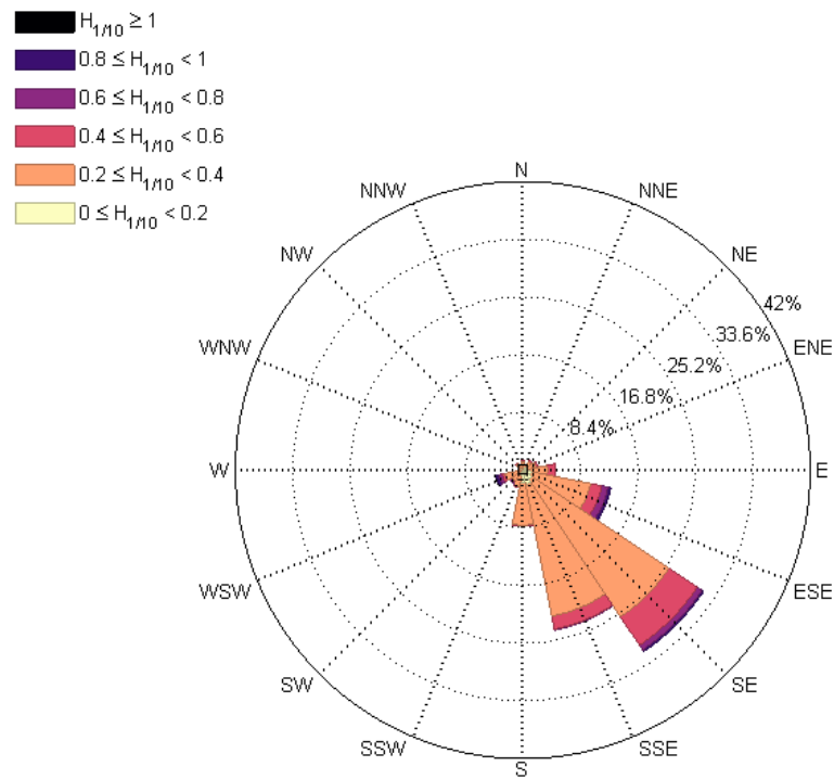
图 4.3.1-9 2019年7月 H1/10 波高波向分级玫瑰图
