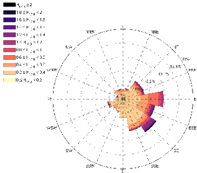
图 4.3.1-11 2019 年 9 月 H1/10 波高波向分级玫瑰图
