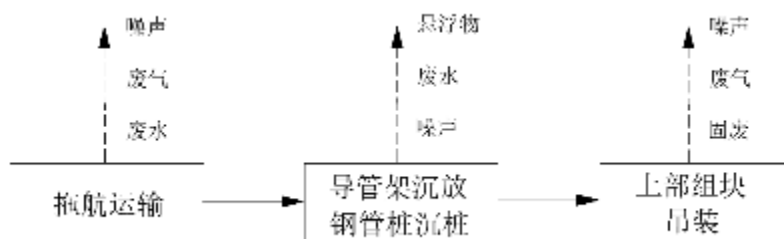
图 3.2.1-2 海上升压站施工主要工序及产污环节
