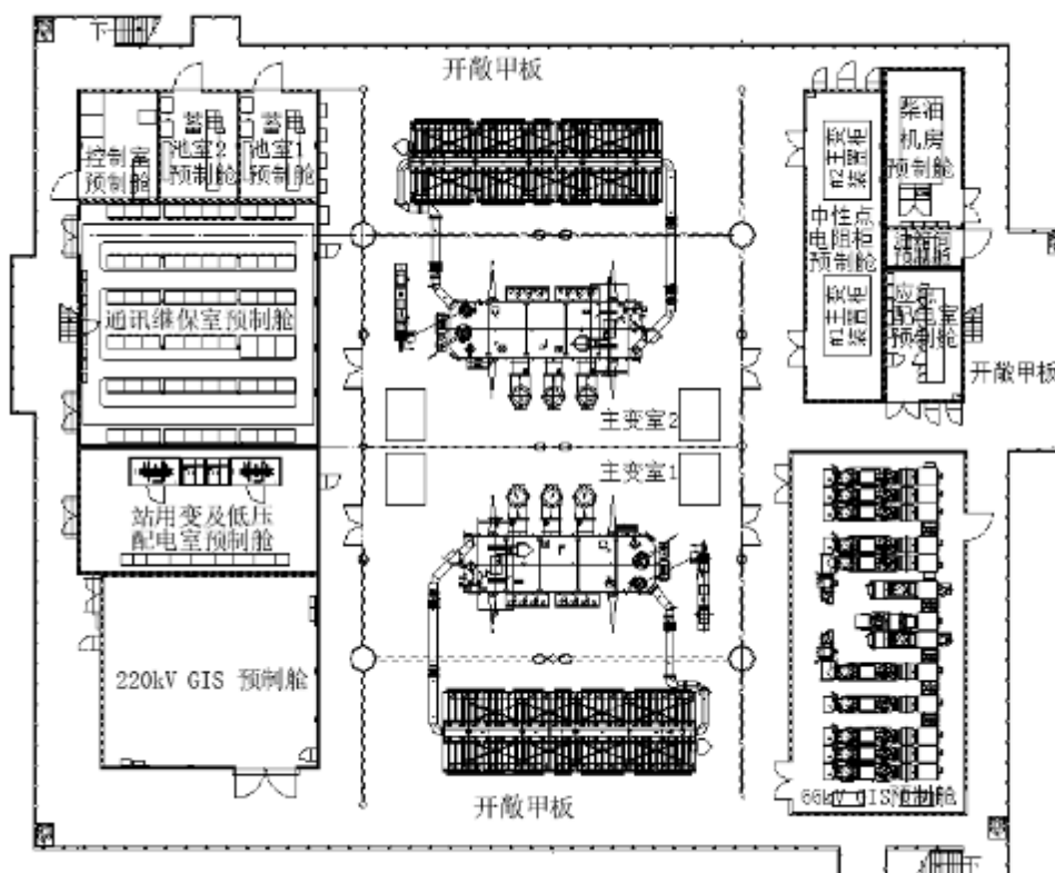
海上升压站二层平面布置示意图
