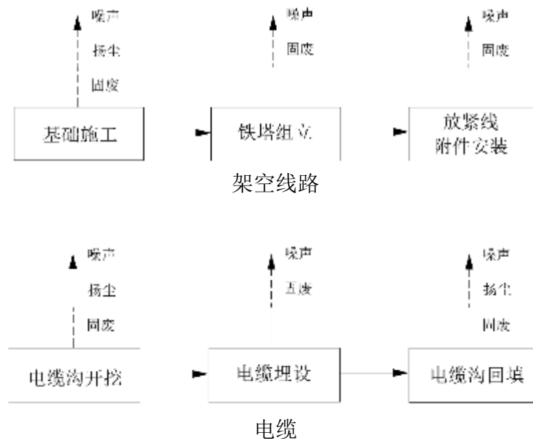
图 3.2.1-4 陆域线路施工工序及产污环节
