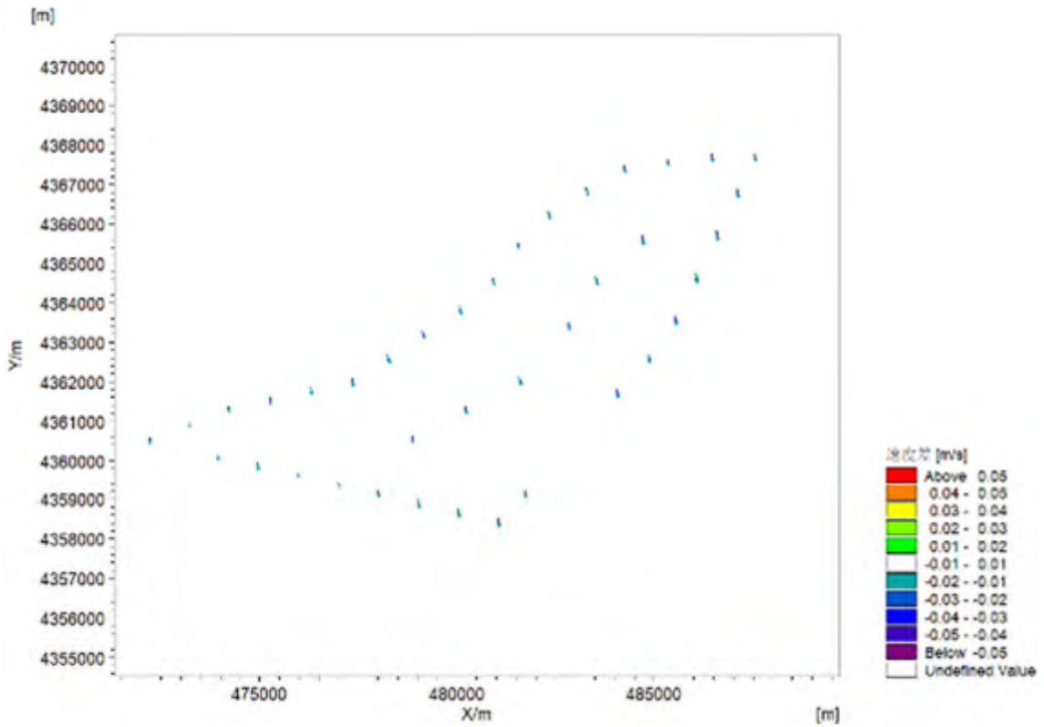
图 5.1.5-2 风电场建成前后工程海域落急流速差值图
