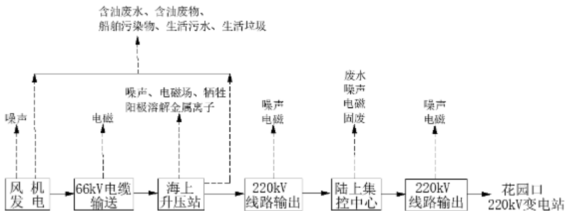
图 3.2.1-6 项目运营期产污环节
