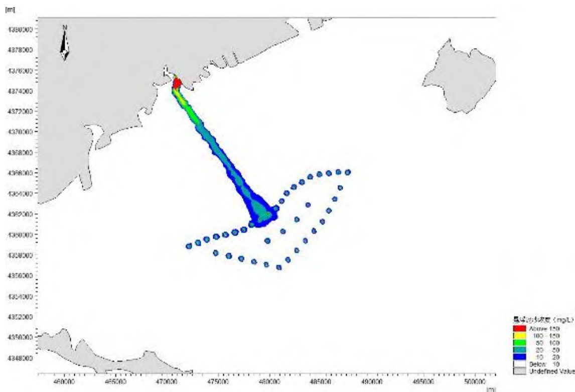
图 5.3.1-2 电缆沟施工期各典型点悬浮物扩散最大影响范围
