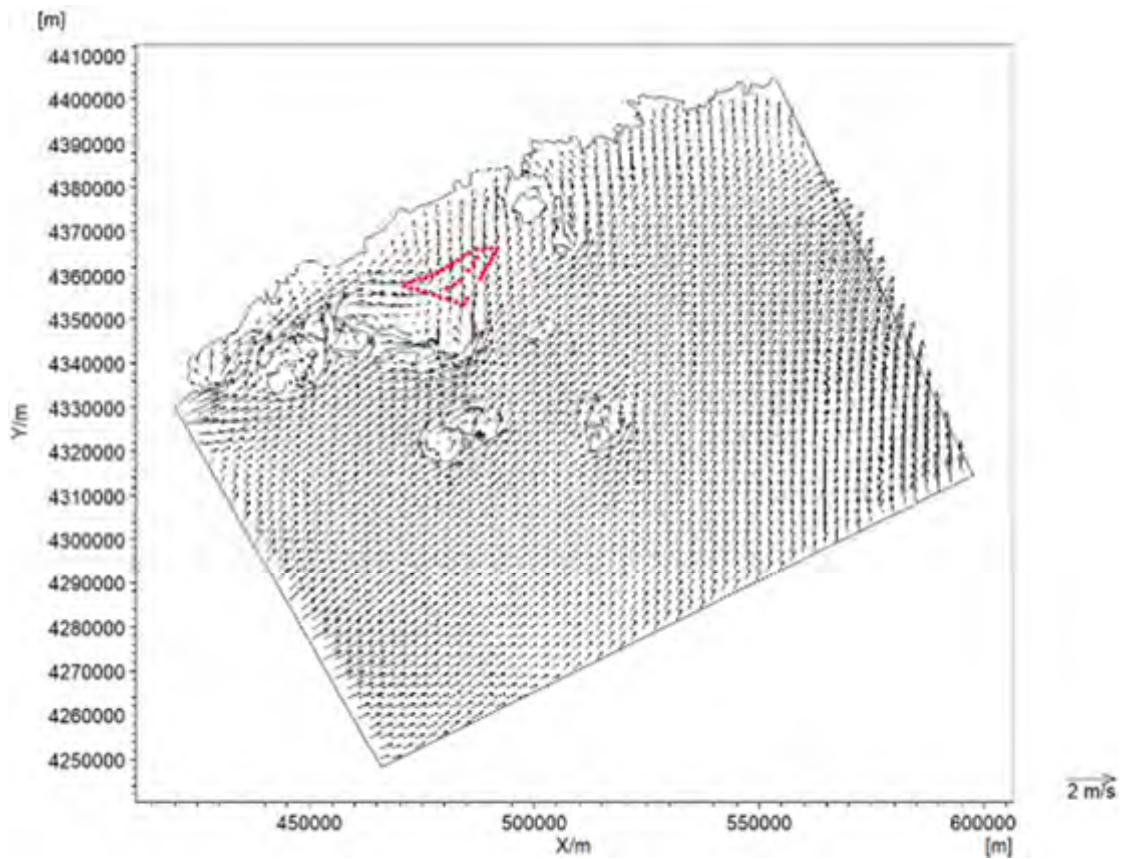
图 5.1.3-1 工程前大范围大潮涨急流场图
