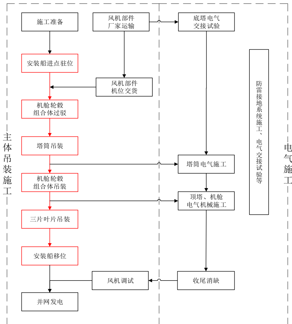
图 3.1.5-4 风机安装施工流程图
