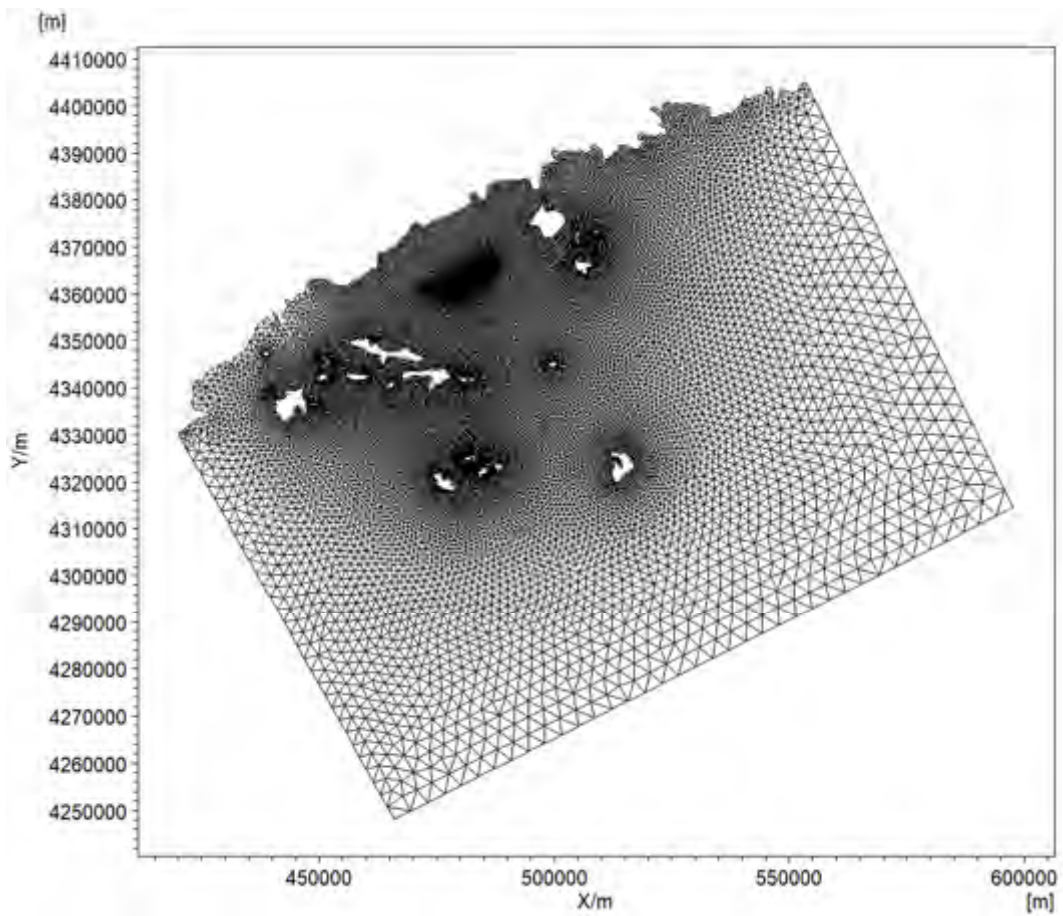
图 5.1.1-2 数值模型计算网格图
