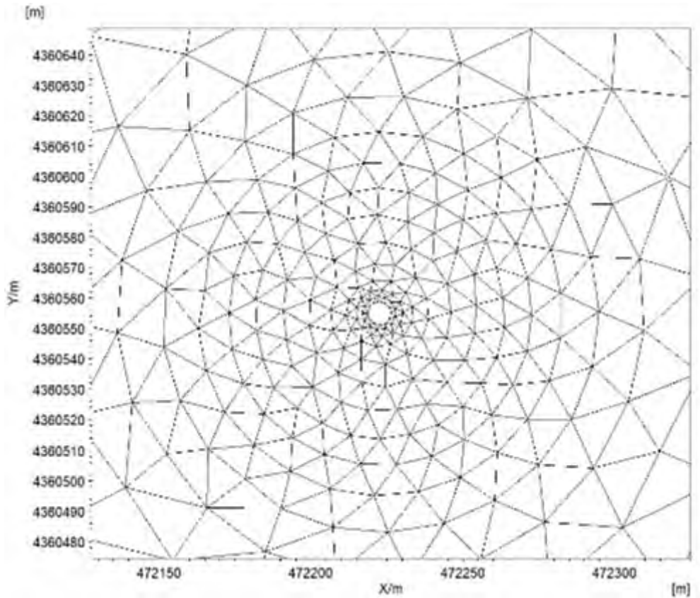
图 5.1.1-4 风电场桩基附近局部网格图
