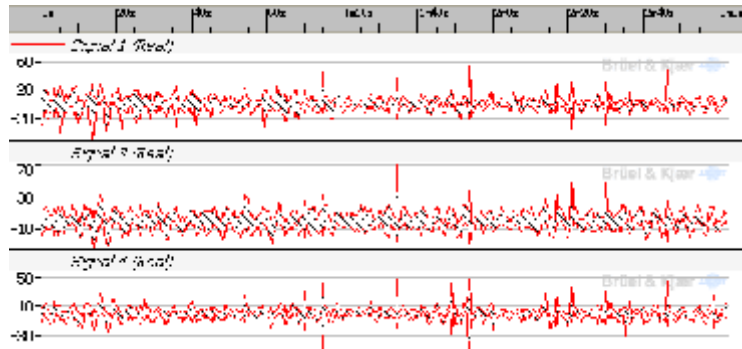
图4.3.9-17 站点 8 水听器在 1m、5m、10m 处所测时域图
