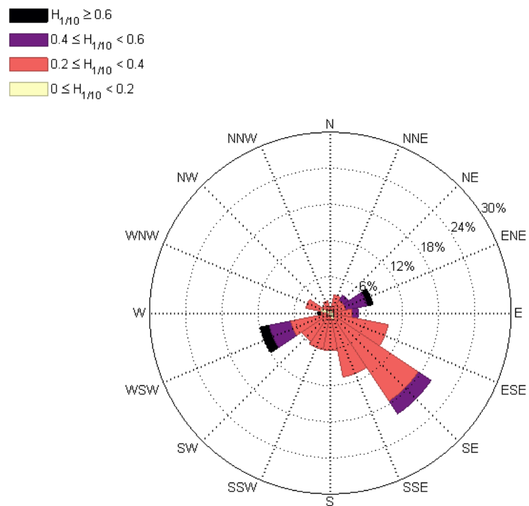
图 4.3.1-8 2019 年 6 月 H1/10 波高波向分级玫瑰图
