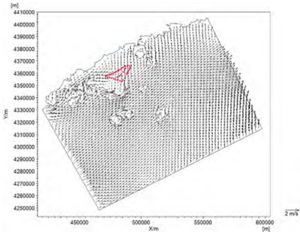
图 5.1.4-1 工程后大范围涨急流场图
