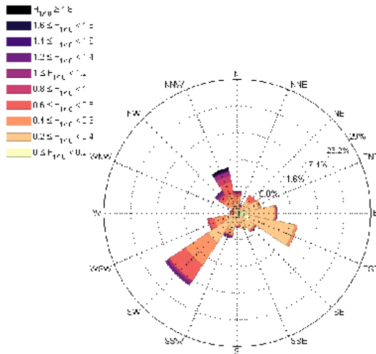
图 4.3.1-12 2019 年 10 月 H1/10 波高波向分级玫瑰图
