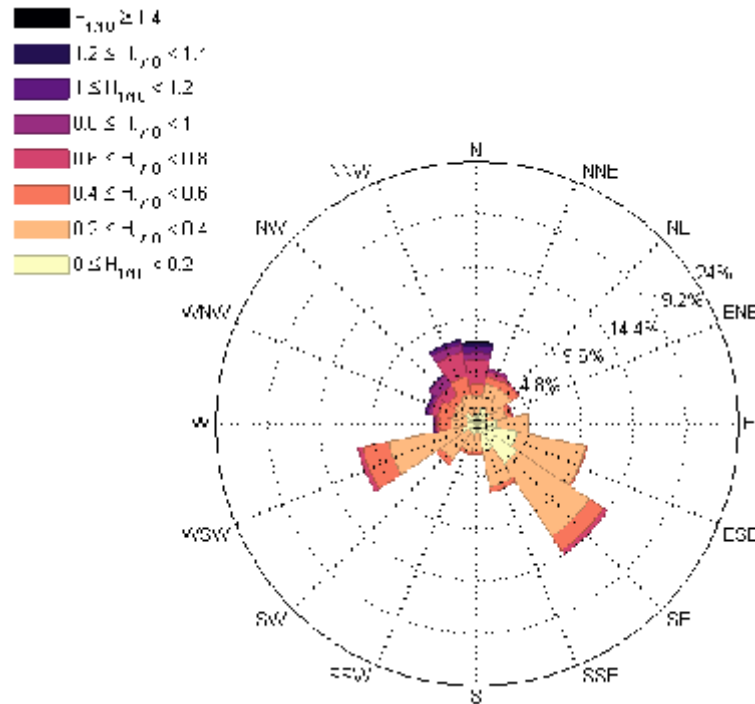
图 4.3.1-17 2020 年 3 月 H1/10 波高波向分级玫瑰图
