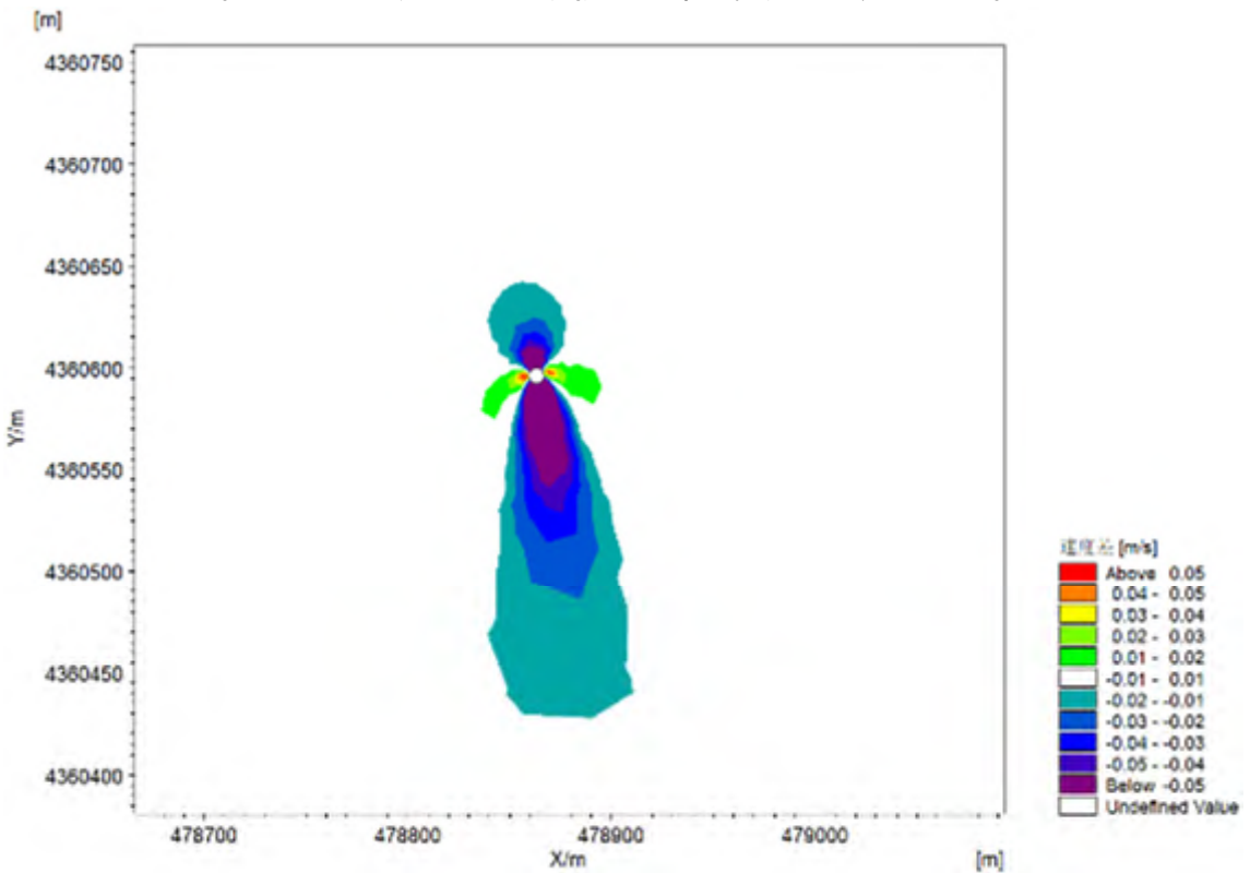
图 5.1.5-3 风电场建成前后桩基局部涨急流速差值图
