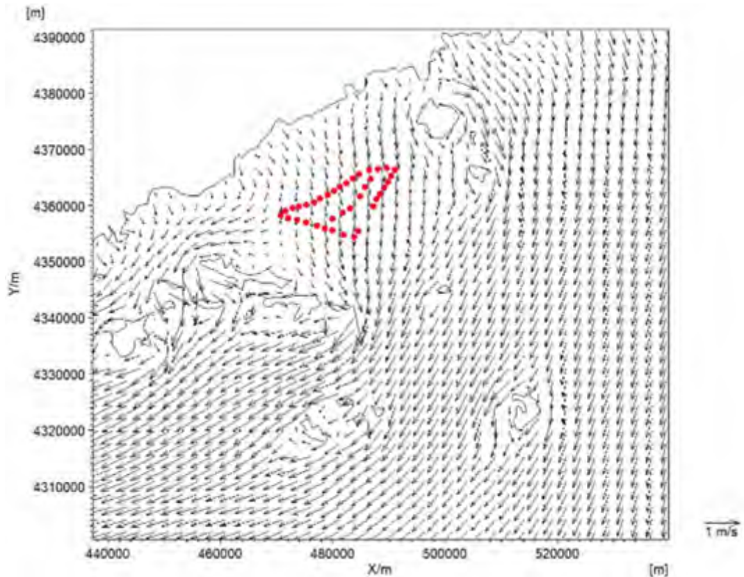
图 5.1.3-4 风电场附近海域大潮落急流场图
