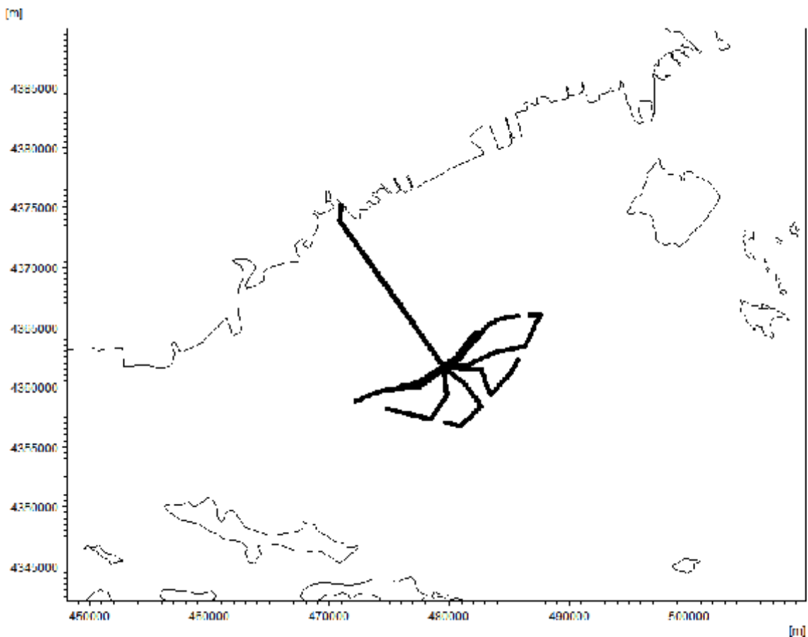
图 5.3.1-1 施工期海缆路由悬浮物扩散排放源示意图
