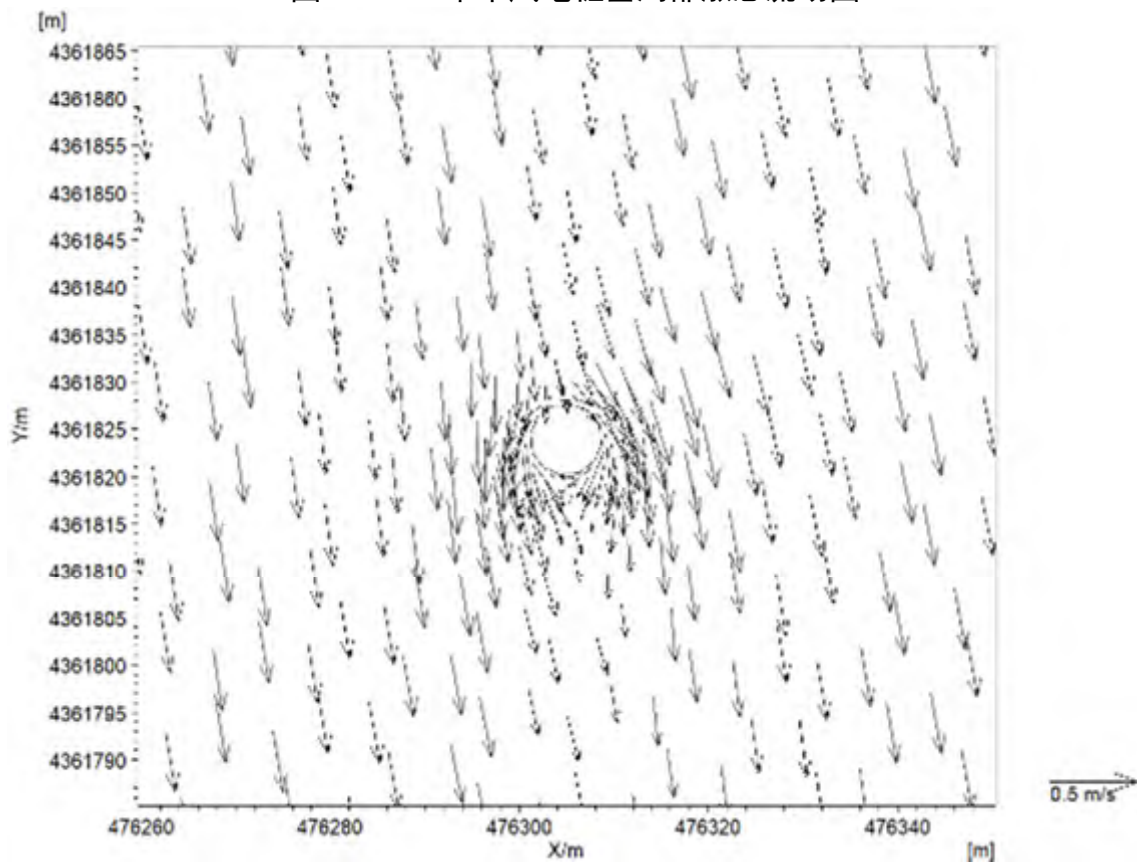
图 5.1.4-4 单个风电桩基局部落急流场图
