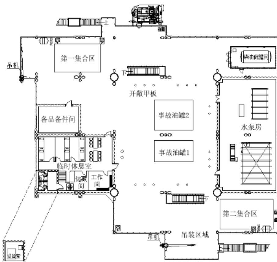
海上升压站一层平面布置示意图
