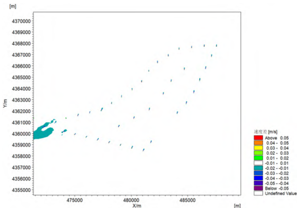
图 5.1.5-1 风电场建成前后工程海域涨急流速差值图
