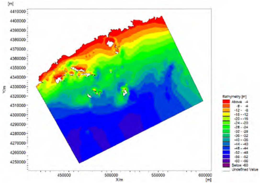
图 5.1.1-1 数值模型计算范围及水深图
