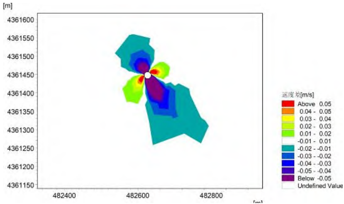
图 5.1.5-4 风电场建成前后桩基局部流速差值图
