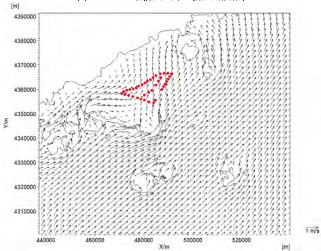
图 5.1.3-3 风电场附近海域大潮涨急流场图
